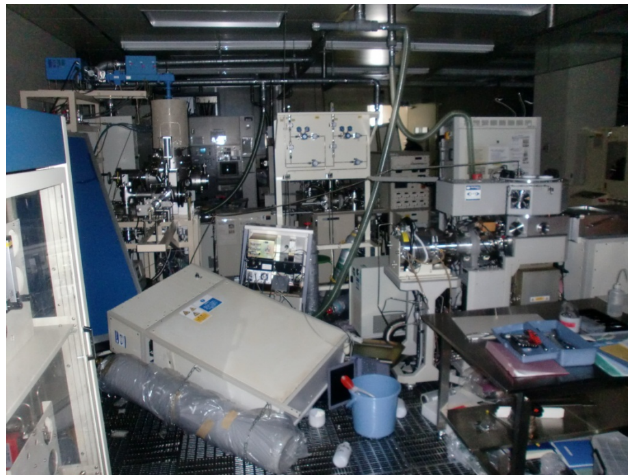
↑周辺装置が横倒しになり、真空ポンプや真空配管が破損した別のDRIE装置
