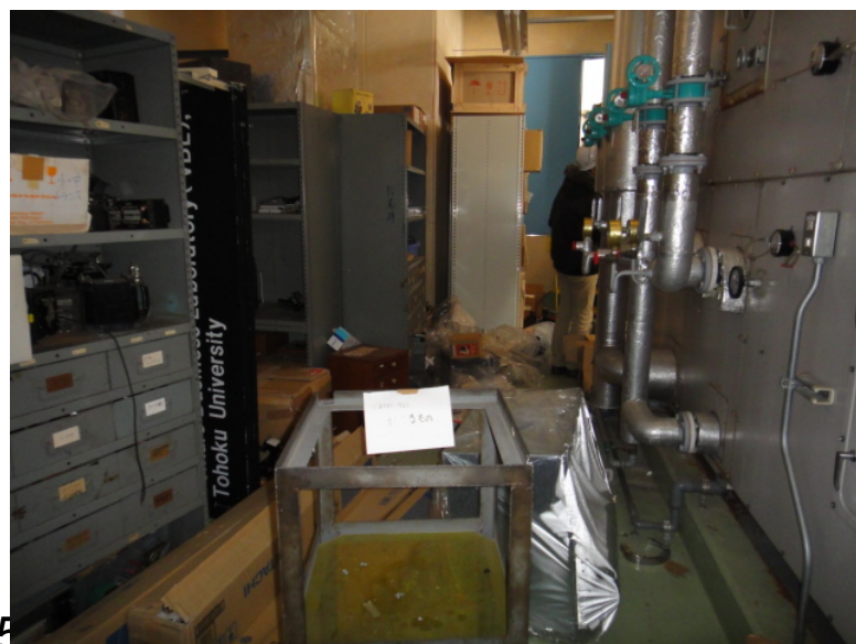
← 空調機と熱交換器のパイプが破損して、水漏れが発生 塩ビの長くて細い空気抜き管が破損して、水漏れが発生
